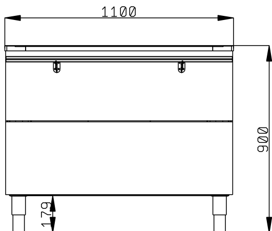
Alzado
